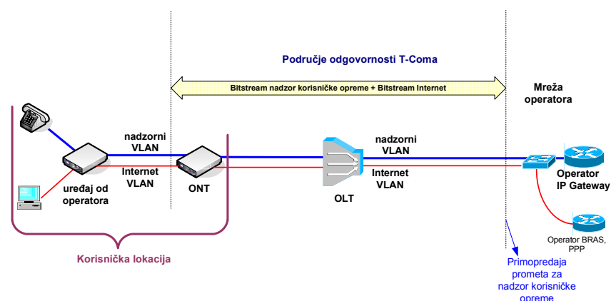
Slika 2227. Veleprodajni širokopojsni pristup za pružanje usluge nadzora korisničke opreme preko FTTH pristupa (GPON) na OLT razini
