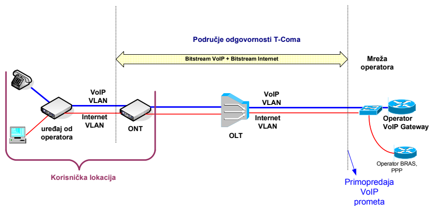
Slika 1417. Veleprodajni širokopojasni pristup za pružanje VoIP usluge preko FTTH pristupa (GPON) na OLT razini
