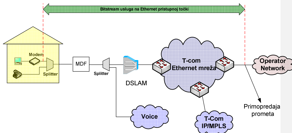
| Slika 4013. Veleprodajni širokopolasni pristup za pružanje VoIP usluge na Ethernet razini u slučaju kada krajnji korisnik ostvaruje osnovni pristup mreži putem usluge T-Coma
