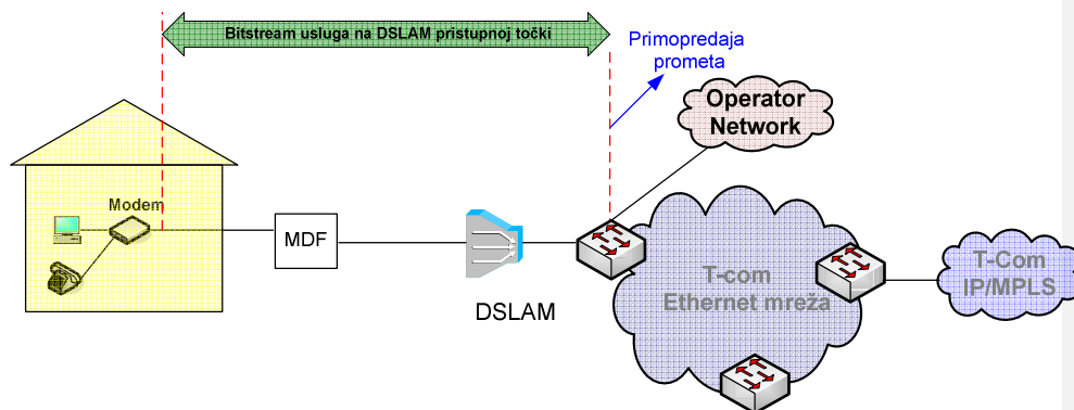
Slika 6. Veleprodajni širokopolasni pristup za pružanje Internet usluge na DSLAM razini u slučaju kada Krajnji korisnik ostvaruje Osnovni pristup mreži putem usluge T-Coma
