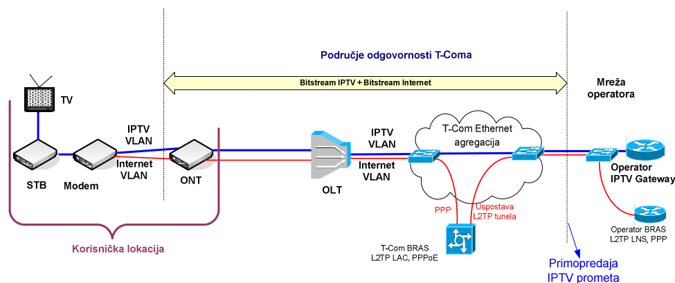
Slika 4822. Realizacija posebnog virtualnog kanala za IPTV uslugu preko FTTH pristupa (GPON)
