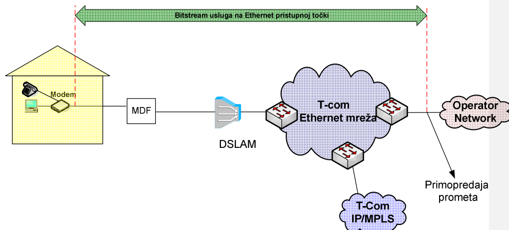
| Slika 4114. Veleprodajni širokopolasni pristup za pružanje VoIP usluge na Ethernet razini u slučaju kada krajnji korisnik ostvaruje osnovni pristup mreži putem usluge Operatora korisnika
