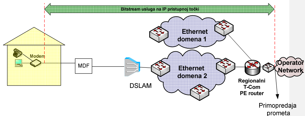
Slika 4215. Veleprodajni širokopojasni pristup za pružanje VoIP usluge na IP razini u slučaju kada Krajnji korisnik ostvaruje Osnovni pristup mreži putem usluge T-Coma
