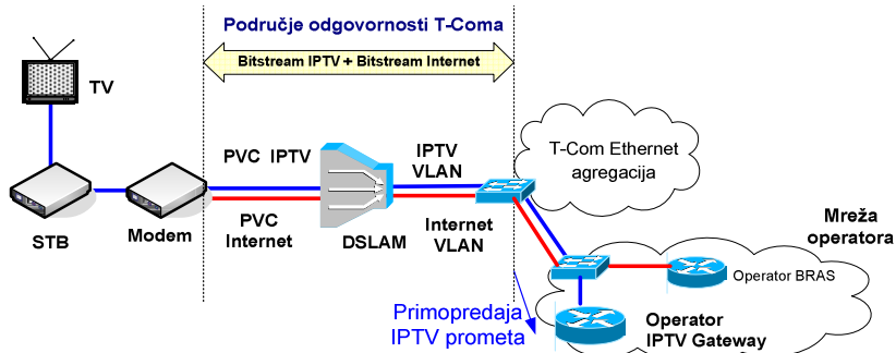
Slika 26. Veleprodajni širokopojasni pristup za pružanje IPTV usluge preko ADSL/VDSL pristupa na DSLAM razini
