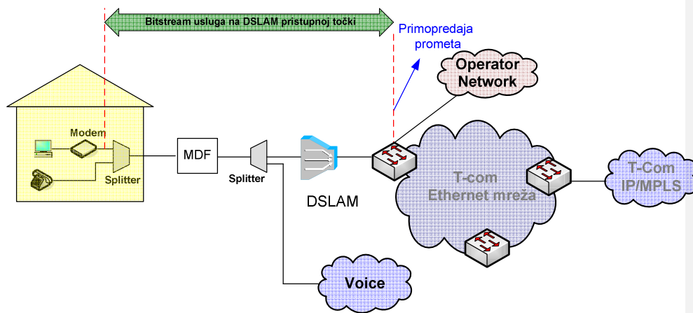
Slika 6. Veleprodajni širokopolasni pristup za pružanje Internet usluge na DSLAM razini u slučaju kada Krajnji korisnik ostvaruje Osnovni pristup mreži putem usluge T-Coma
