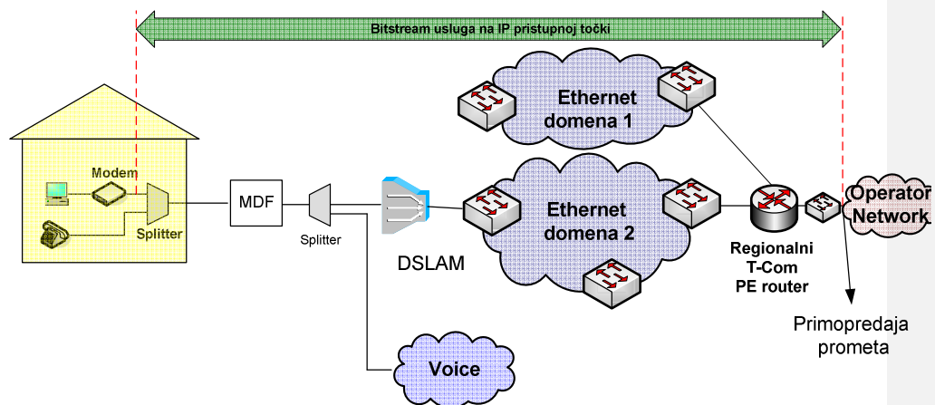
Slika 4215. Veleprodajni širokopojasni pristup za pružanje VoIP usluge na IP razini u slučaju kada Krajnji korisnik ostvaruje Osnovni pristup mreži putem usluge T-Coma
