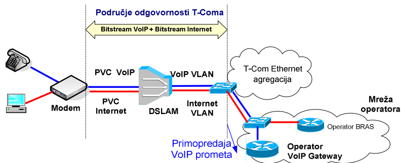
Slika 18. Veleprodajni širokopojasni pristup za pružanje VoIP usluge preko ADSL/VDSL pristupa na DSLAM razini
