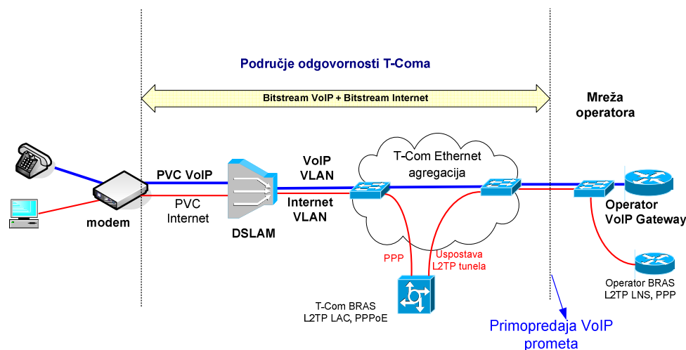
Slika 811. Realizacija posebnog virtualnog kanala za VoIP uslugu preko ADSL/VDSL pristupa (kod VDSL pristupa između modema i DSLAM-a koristi se odgovarajući VLAN)
