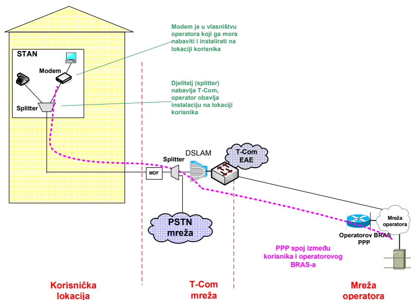
Slika 8. Način realizacije Veleprodajnog širokopojasnog pristupa za pružanje Internet usluge na DSLAM razini
