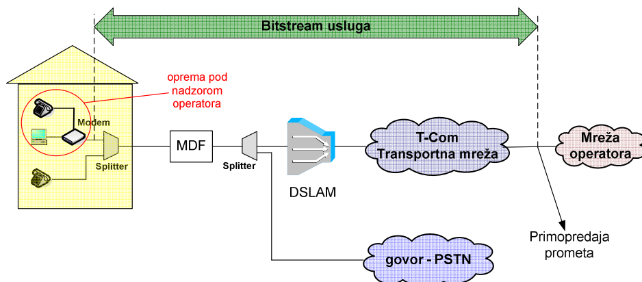
Slika 69. Koncept posebnog virtualnog kanala za VoIP uslugu u slučaju kada Krajnji korisnik ostvaruje Osnovni pristup mreži putem usluge T-Coma
