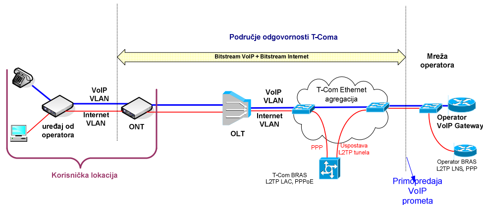
Slika 912. Realizacija posebnog virtualnog kanala za VoIP uslugu preko FTTH pristupa (GPON)
