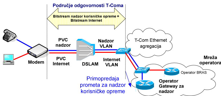
Slika 28. Veleprodajni širokopolasni pristup za pružanje usluge nadzora korisničke opreme preko ADSL/VDSL pristupa na DSLAM razini
