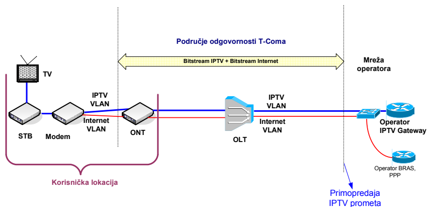
Slika 2425. Veleprodajni širokopojasni pristup za pružanje IPTV usluge preko FTTH pristupa (GPON) na OLT razini
