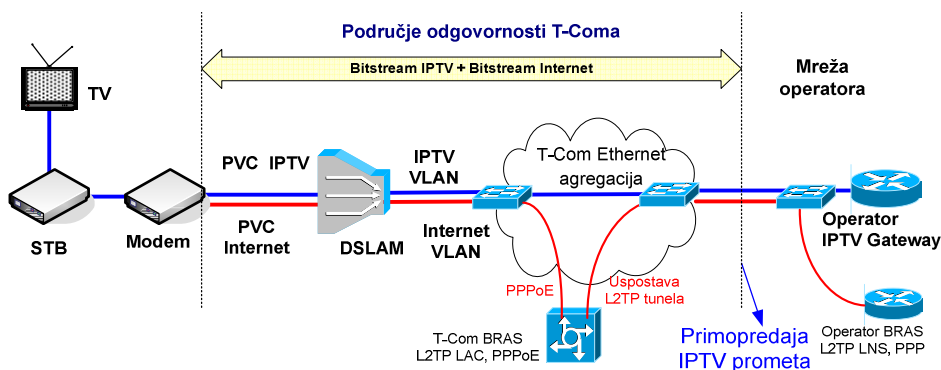
| Slika 1721. Realizacija posebnog virtualnog kanala za IPTV uslugu preko ADSL/VDSL pristupa (kod VDSL pristupa između modema i DSLAM-a koristi se odgovarajući VLAN)
