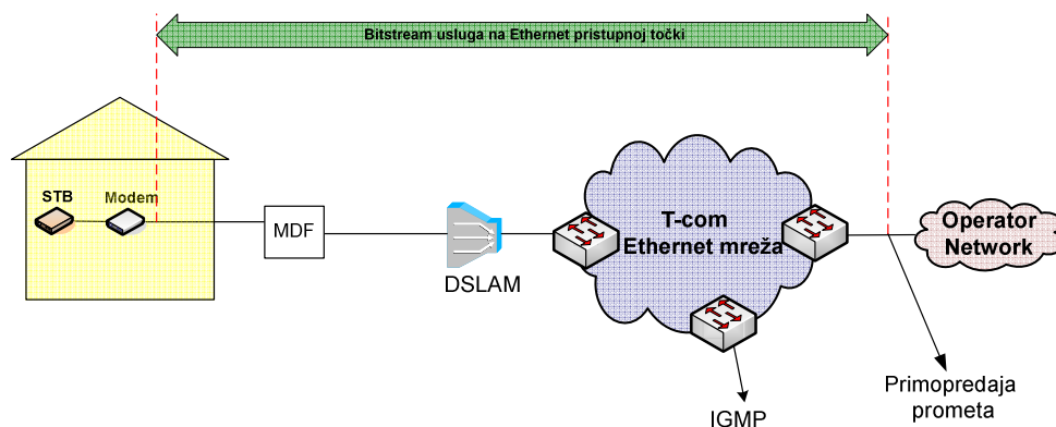
Slika 1923. IPTV usluga na Ethernet razini putem ADSL/VDSL tehnologije u slučaju kada Krajnji korisnik ostvaruje Osnovni pristup mreži putem usluge T-Coma
